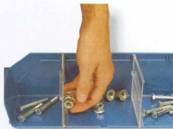
schalenförmige Trennplatten erleichtern das Entnehmen der Kleinteile
